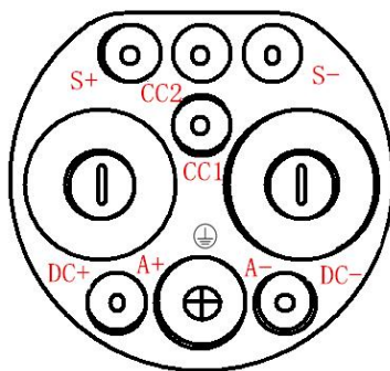
图 1-2 充电插头接口图
