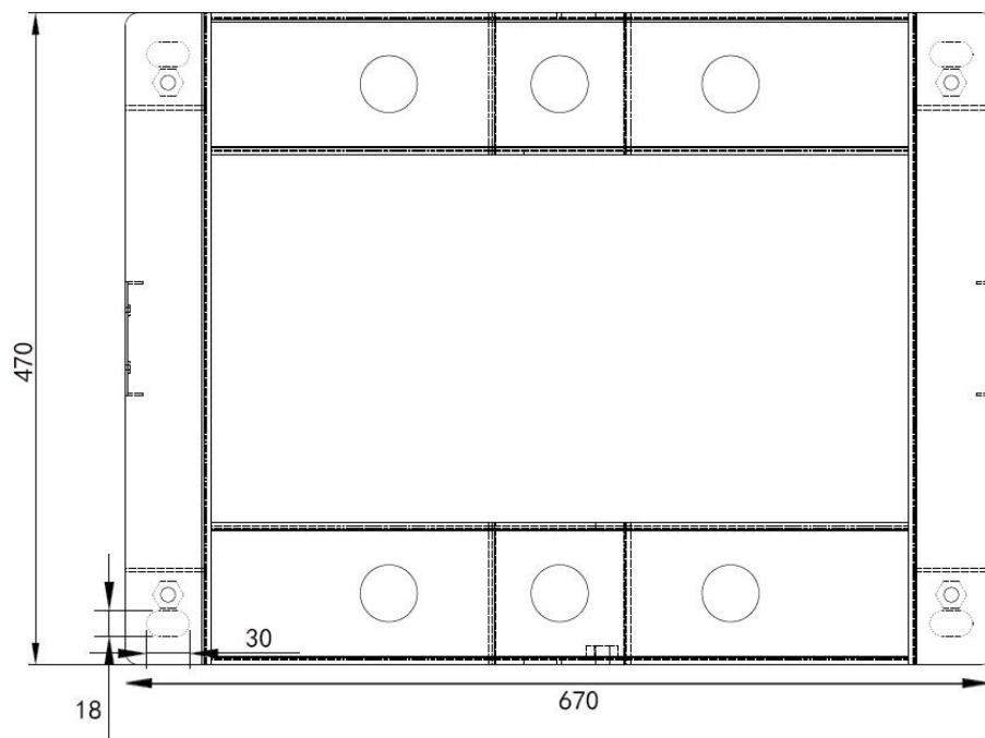
机柜底座俯视图
