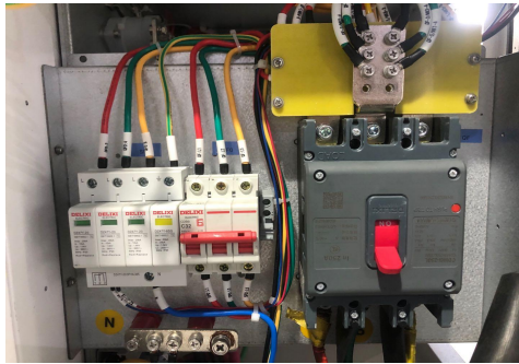
图 3-1 打开前门观察积尘
