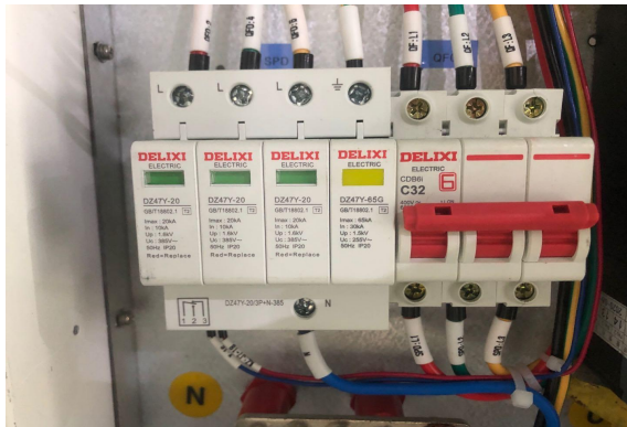
图 3-8 检查浪涌保护器及线路的老化、磨损情况
