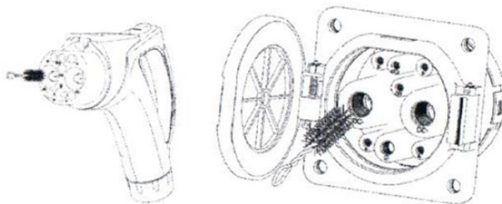
图 3-19 清洁充电枪及插座
