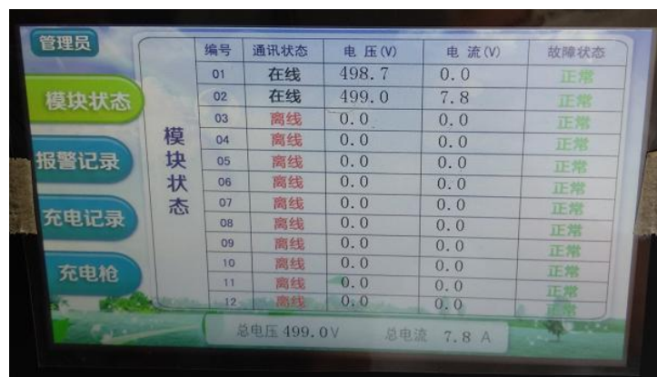
图 2-20 模块状态参数
