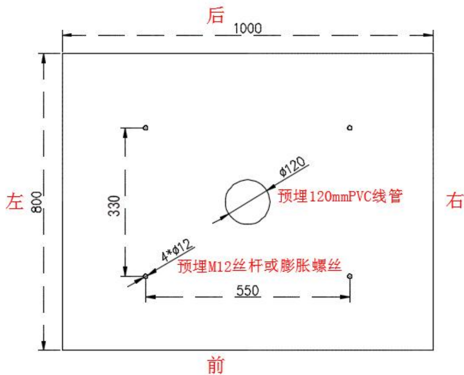
混凝土基础俯视图
